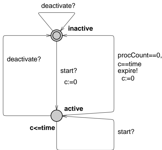
Fig. 10. The Timer automaton.
