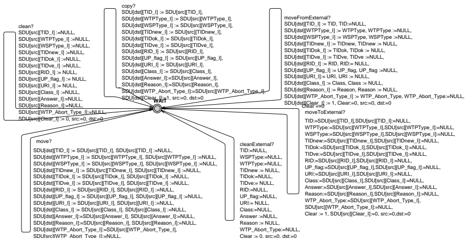
Fig. 9. The Datasstore automaton.
