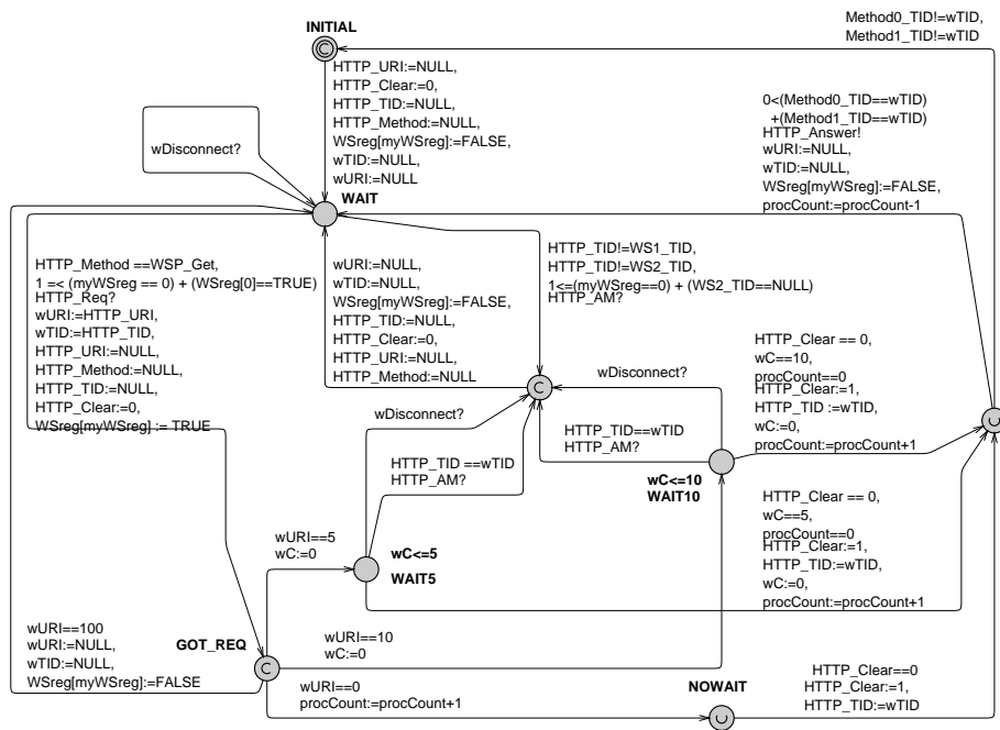
Fig. 15. The HTTP Server automaton.
